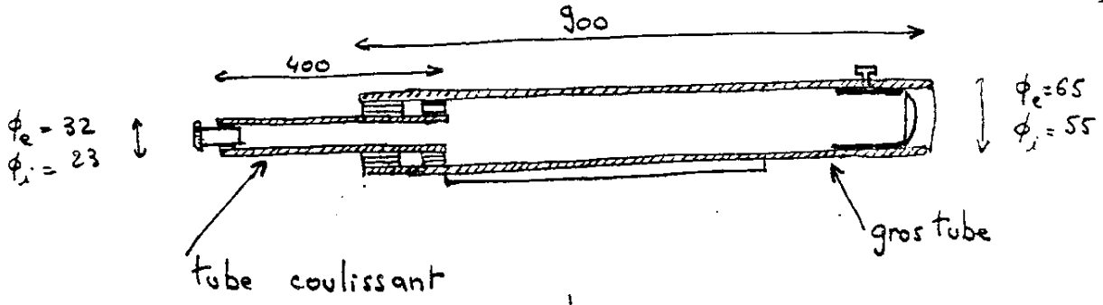
schéma général
